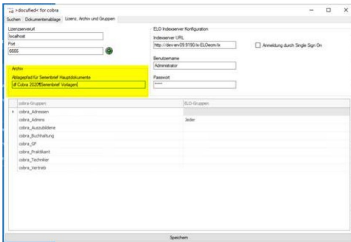
Abbildung 27 - Konfiguration: Ablagepfad für Serienbrief-Hauptdokumente
